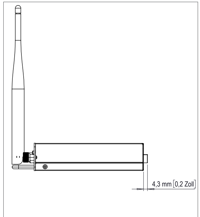
Seitenansicht
