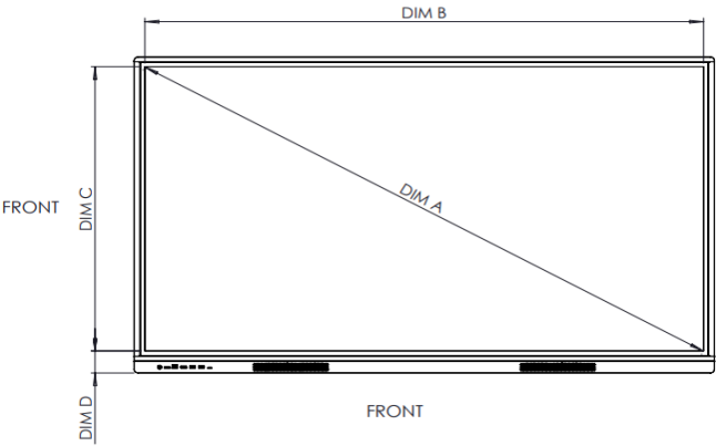
Vorderansicht
