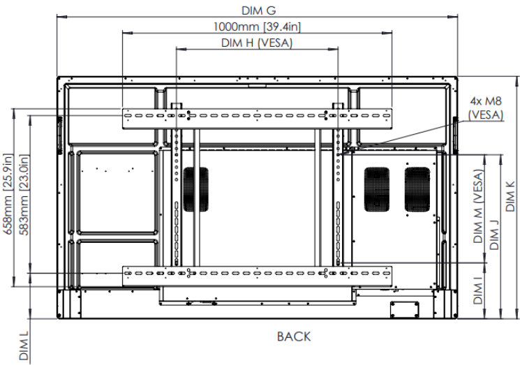
Rückansicht
