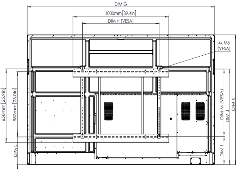
Rückansicht
